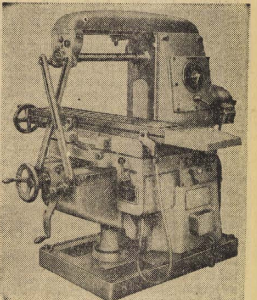
Az ME 1000 egyetememes marógép, a gyár egyik kitűnő gyártmánya
